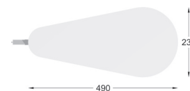
VA 1215 Display shelf "TEAR DROP"
