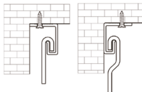
Immagine 3: installazioni a soffitto
