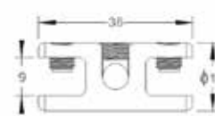
AE-AS/CCV connettore centrale: viene installato nelle aste centrali su strutture multiple
