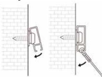
Immagine 1: Installazione muro
